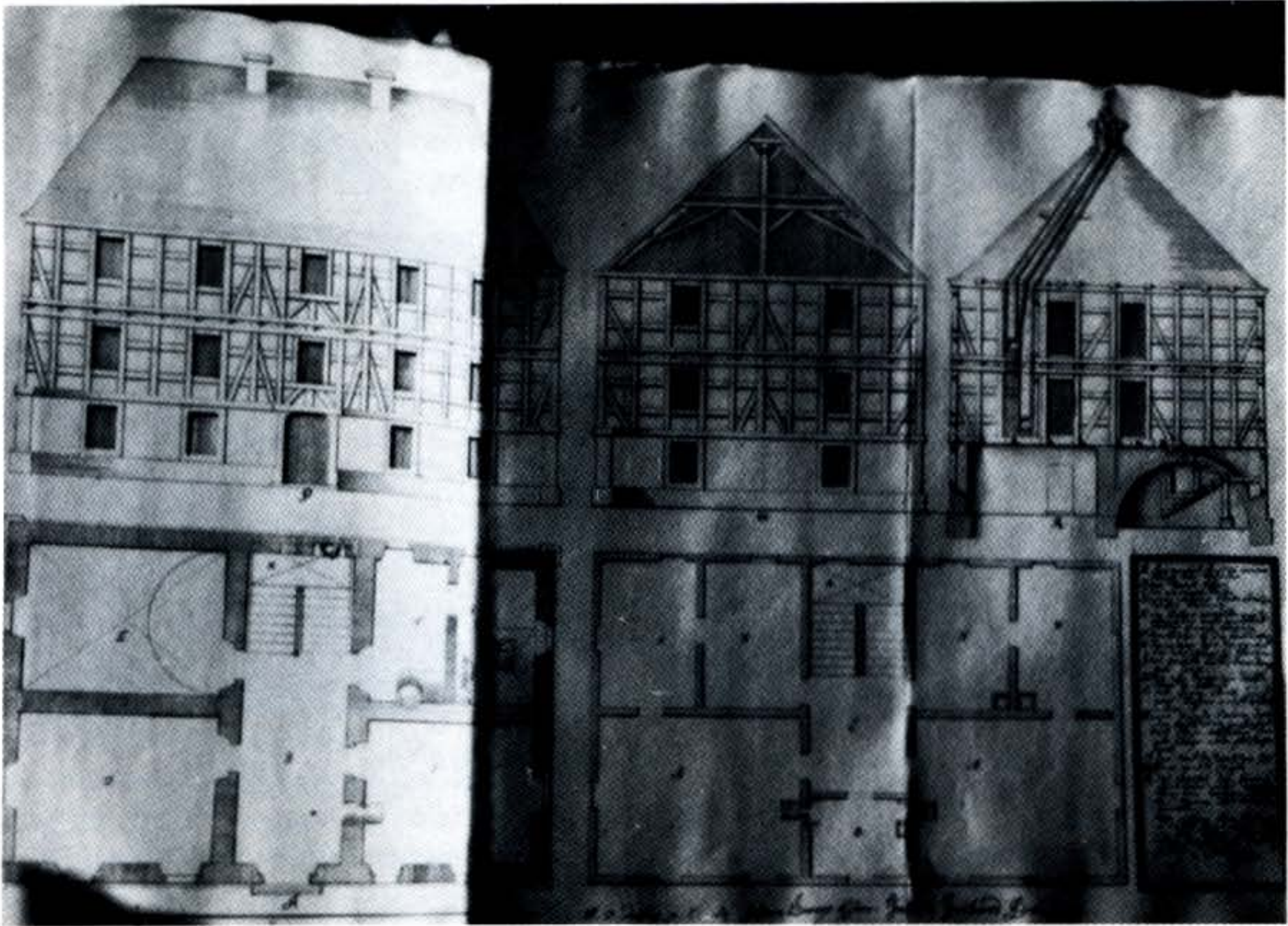
Plan von Baumeister Cöster (letzter Entwurf 1750) für Vogteigebäude Singlis
